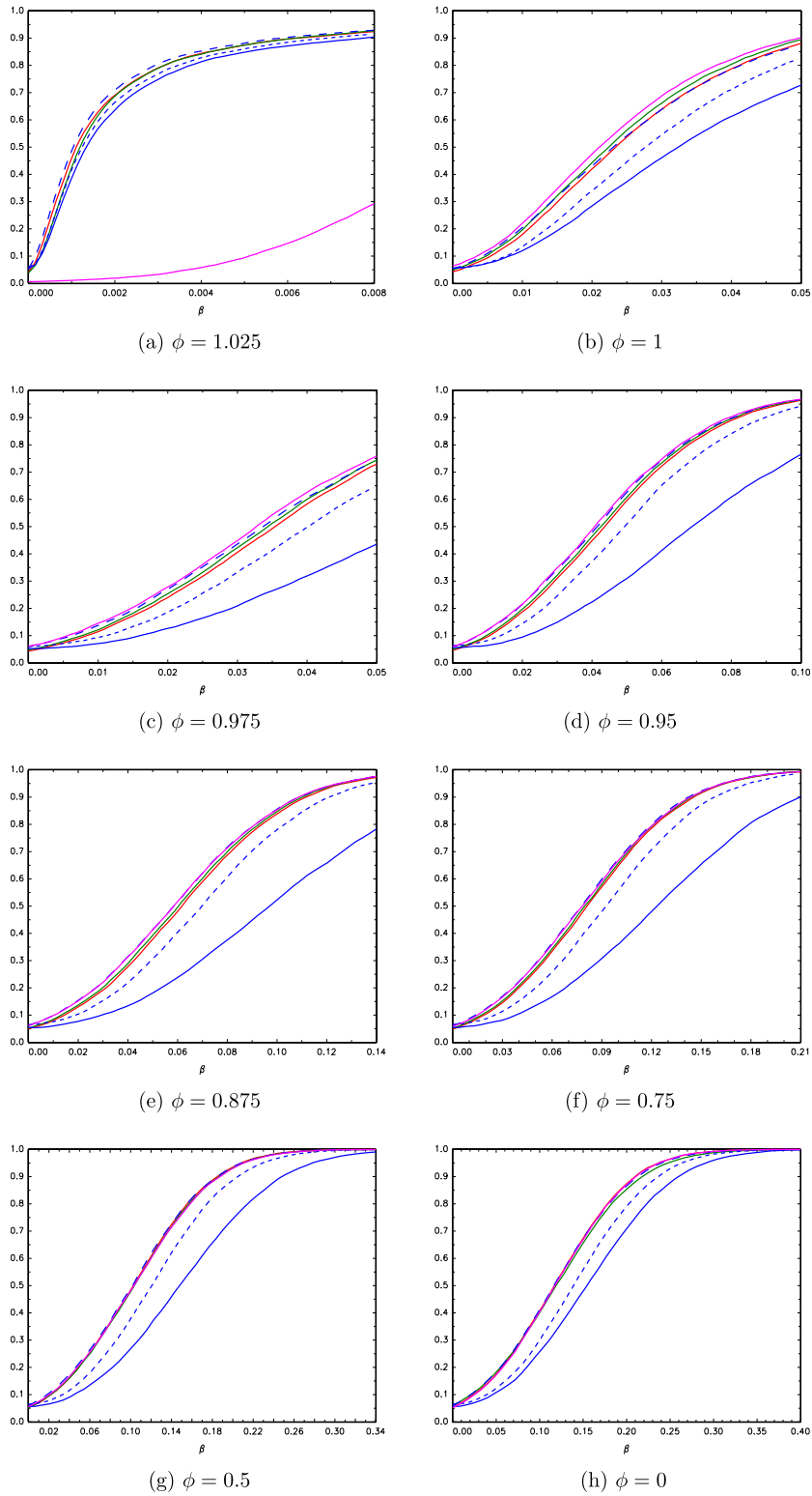
Fig. 4. Finite sample power of nominal 0.05-level tests, T = 200 , \rho_{xy} = 0 ; \tau_{ihyb} : —, Q : —, BD : —, IVX_1 : - - -, IVX_2 : - · - · -, EMW : —.
