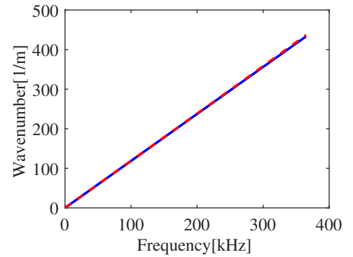
Fig. 4. Dispersion curves for the bar: analytical(-), WFE(- -)
