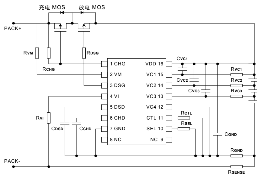
3 串电池连接
