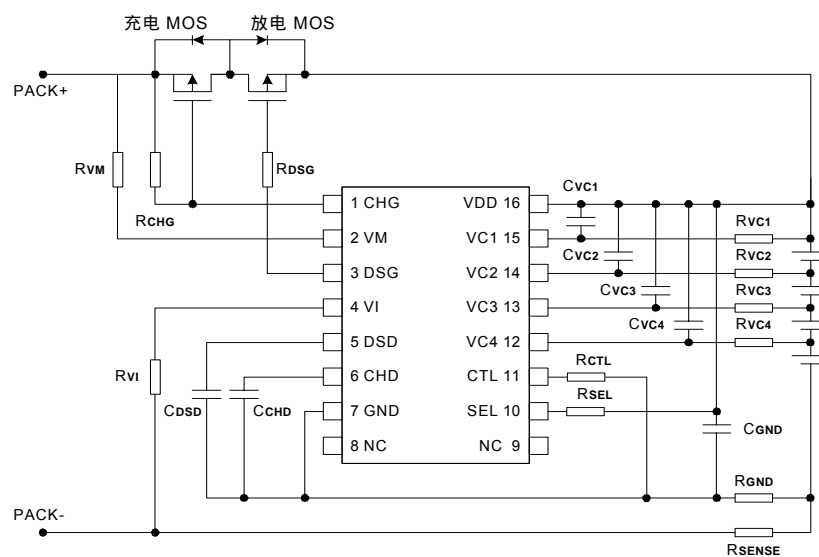
4 串电池连接
