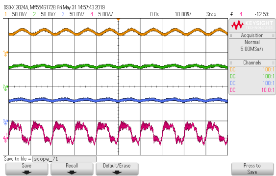
(d) Asymmetrical power flow: 100 Hz ac component at input port
